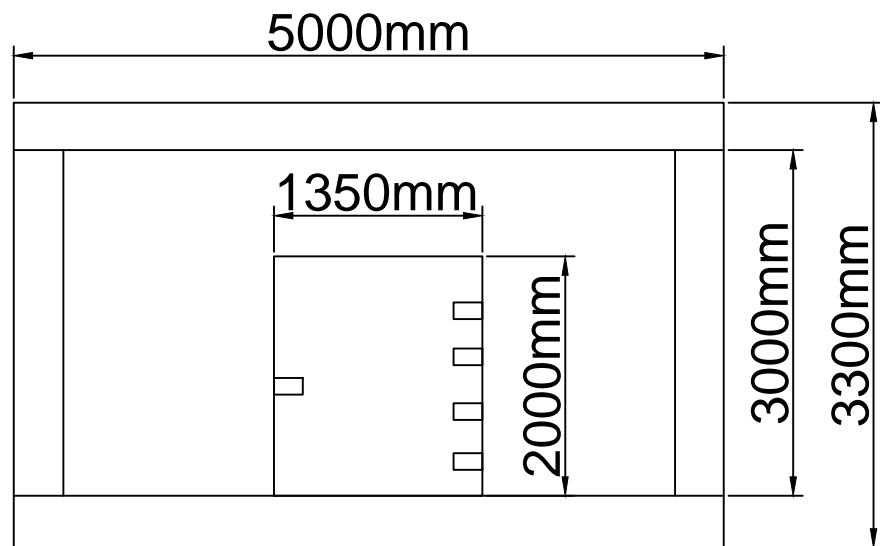
冷凍庫側視圖
