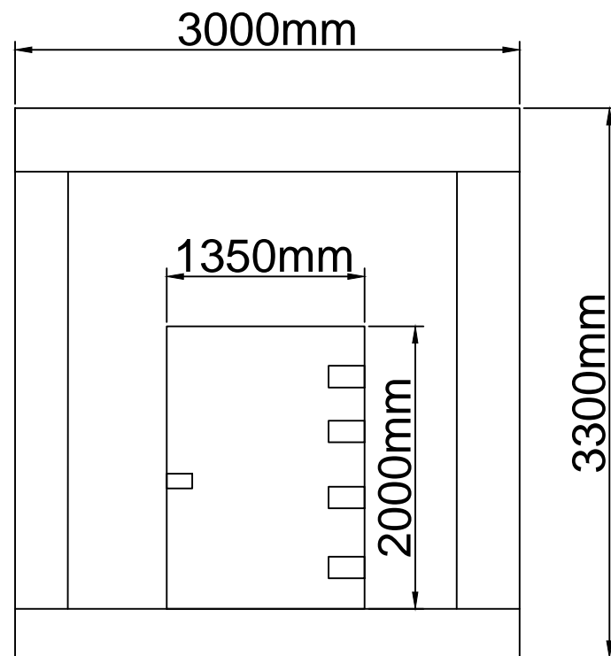
冷凍庫正視圖
